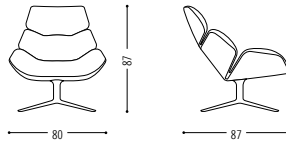
Stuhl mit Holzgestell, nicht stapelbar Chair with wooden frame, non-stackable
