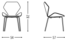
Stuhl mit Metallgestell, stapelbar Chair with metal frame, stackable
